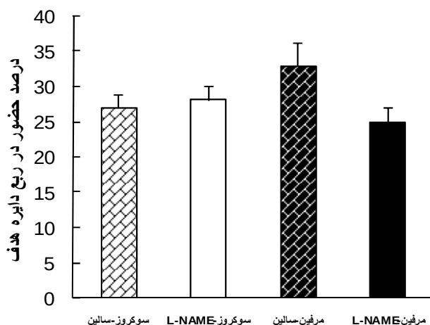
شکل ۴- مقایسه درصد حضور حیوانات در ربع دایره هدف در مرحله Probe trial در گروههای مورد مطالعه ( n = 10-7 )
