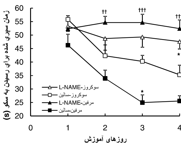
شکل ۱- مقایسه زمان سپری شده برای رسیدن به سکو (Escape latency) در چهار گروه مورد مطالعه در طی روزهای آموزش ( n = 7-10 ) P < 0.05 * نسبت به گروه سوکروز-سالین و P < 0.01 † و P < 0.001 †† نسبت به گروه مرفین-سالین
