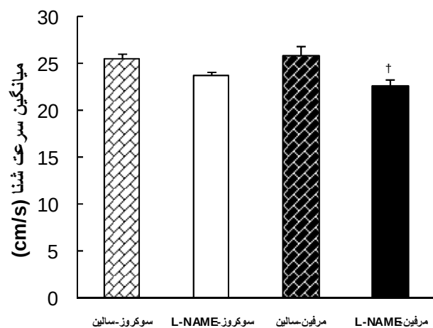
شکل ۳- مقایسه میانگین سرعت شنای حیوانات در چهار گروه آزمایش در طی روزهای آموزش ( n = 10-7 ). P < 0.05 † نسبت به گروه مرفین-سالین
