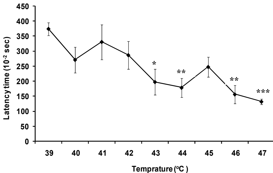
شکل ۱۰-۱ اثر دماهای مختلف در ایجاد درد در مگس سرکه بالغ موتان Vestigial به درد حرارتی. افزایش دما از ۳۹°C تا ۴۷°C باعث کاهش زمان پاسخ مگس بالغ به حرارت (مدت زمان استقرار روی Hot plate) می شود. آستانه پاسخ در دمای ۴۳°C بوده ( p < 0.05 ), بیشترین پاسخ در ۴۷°C می باشد. ( p < 0.001 و p < 0.01 و p < 0.05 در مقایسه با پاسخ جانور در دمای ۳۹°C نتایج به صورت \text{Mean} \pm \text{SEM} ارائه شده است ( n=10 ).
