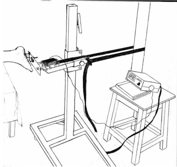
شکل ۱- دستگاه طراحی شده جهت اعمال تحریرات مکانیکی
